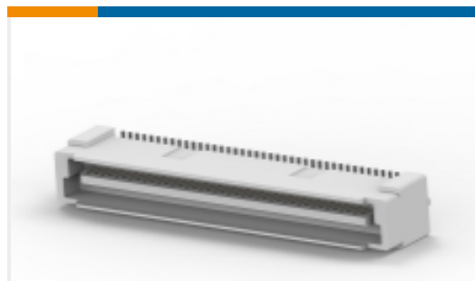
TE 系列/零件编号 5179031-3 0.8FH,P08H.5,080,08/Sn,TU
