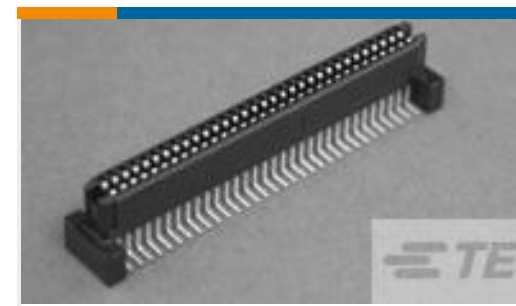
TE 系列/零件编号 1-120529-1 1FHR,64,50A/P,N,C,S11,12
