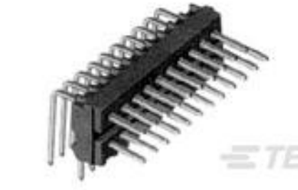
TE 系列/零件编号 6-104118-6 80 SYS 50 HDR DRRA UNSHRD SN
