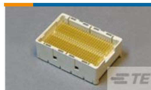
TE 系列/零件编号 1-1761616-2 STEP-Z PLUG 12MM 296P PB ST
