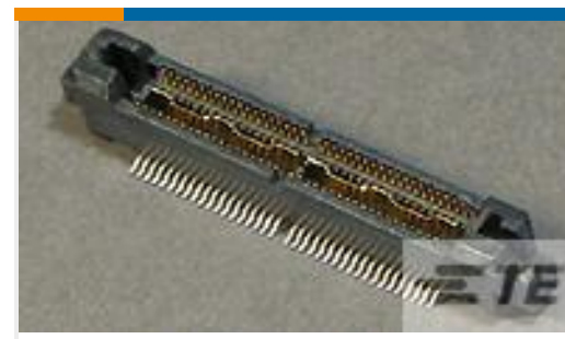
TE 系列/零件编号 5767111-2 MICT,PLG,076,ASY,.025 TAPE PKG
