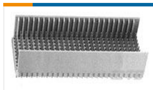
TE 系列/零件编号5646357-9 2MM HM ASY,T-B,HDR,10R,250,LUB
