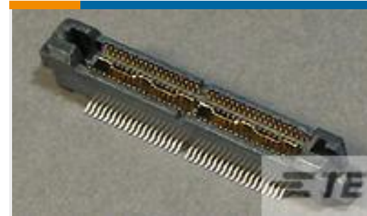
TE 系列/零件编号 5767118-9 MICT,PLG,076,ASY,.025,TAPE PKG
