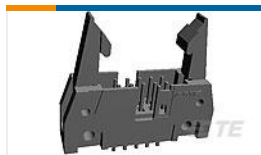
TE 系列/零件编号499374-2 014 UNIV HDR SP 4S 30DP STD L2
