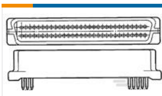
TE 系列/零件编号6-5173280-4 AMPLIMITE.050 CAP ASS'Y (V) 60
