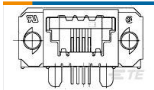
TE 系列/零件编号1-1761199-1 4 POSN SE SDL RCPT W/BDLK
