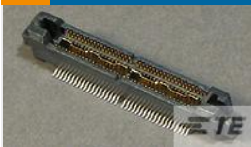
TE 系列/零件编号 5767057-2 MICT,495,PLUG,076,PDNI
