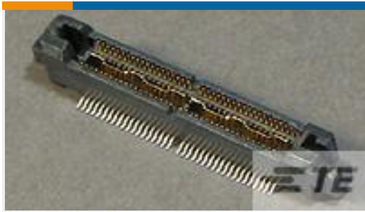
TE 系列/零件编号 2149084-9 MICT,PLG,076,ASY,.025 TAPE CAP
