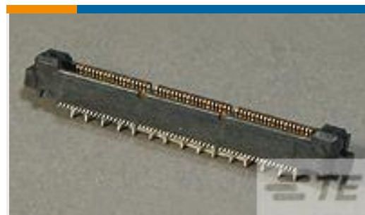
TE 系列/零件编号 5767116-3 MICT,260PLG,114,ASY,.025,AUPLT
