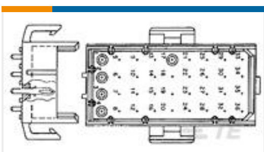
TE 系列/零件编号640497-4 02P MR HDR ASSY V0 RED
