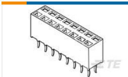
TE 系列/零件编号215308-7 2X 7P HV100 REC CON. TE, 7.0MM, TIN
