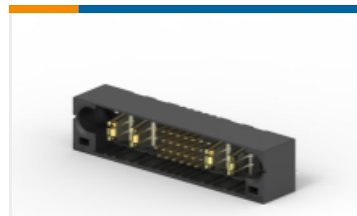
TE 系列/零件编号4-6600333-5 MBXL VERT HDR 2ACP+24S+2ACP
