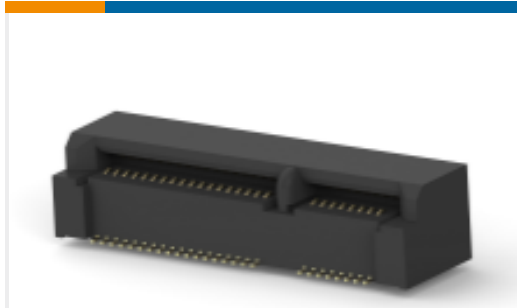
TE 系列/零件编号1759547-1 mSATA/mini PCI-E 7H G/F
