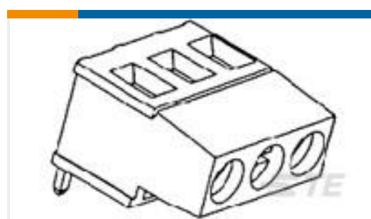
TE 系列/零件编号282862-2 TERMI-BLOK PCB MOUNT 180 2P.5
