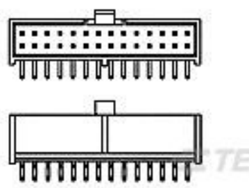
TE 系列/零件编号1-1888292-3 FPH-2002G=FLXPAC HDR P 20 RA LF
