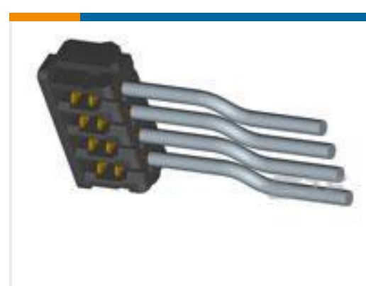
TE 系列/零件编号 2-179694-2 2MM CT MT REC ASSY 2P GRAY
