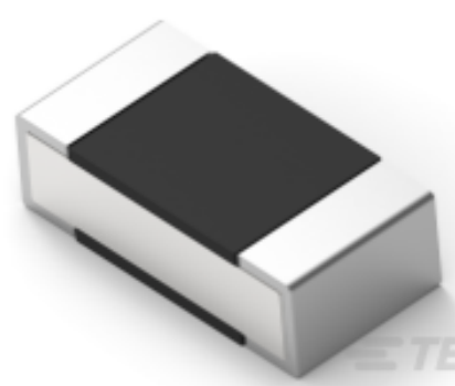
TE 系列/零件编号7-2176304-8 RP 1E 0.1W 63R4 0.1% 25PPM 5K RL
