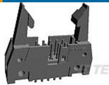
TE 系列/零件编号3-5499206-1 A/L UNIV HDR 60P VERT LG LAT BLUE
