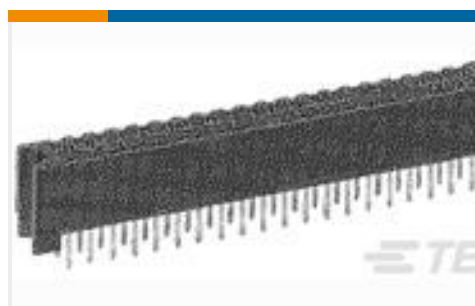
TE 系列/零件编号5-534972-3 50 MODII VRT 2PC DR CE 100CL, RoHS
