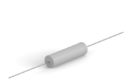
TE 系列/零件编号7-2176414-0 7W STD M/OX 5% 15K
