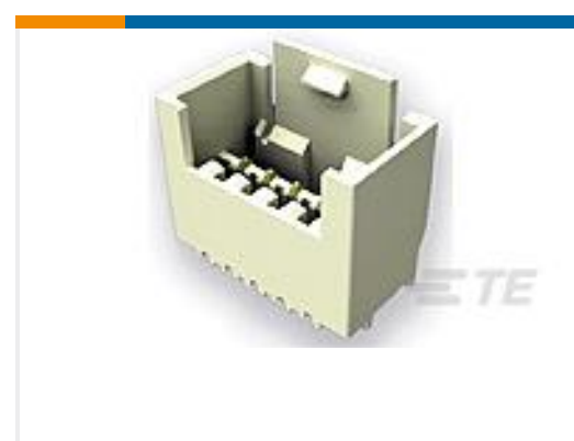
TE 系列/零件编号 1-1971837-0 10P,RAST 2.5 Tab Header,Ex- Locking, THV
