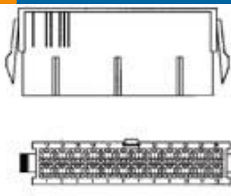
TE 系列/零件编号1-1586861-2 12P PM PLUG VAL-U-LOK PM GW
