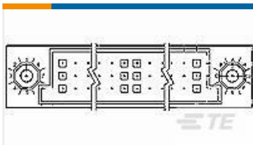
TE 系列/零件编号5532447-5 ASSY,PIN,VERTICAL,HDI,LEAD-FRE
