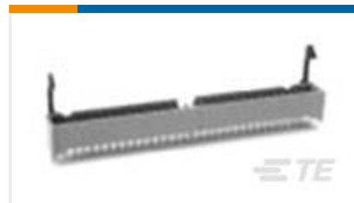
TE 系列/零件编号3-1761711-5 IDC LOW PRO HDR 50P VERT LG LA
