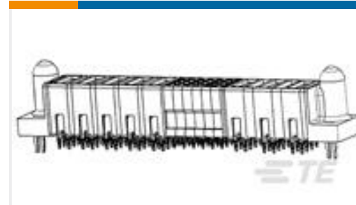
TE 系列/零件编号1892430-4 MBXL VERT RCPT 6P+24S+6P
