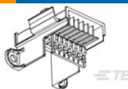
TE 系列/零件编号293039-2 7 POS. F.F. TAB HSG MOTOR MOUNT WATER-PR
