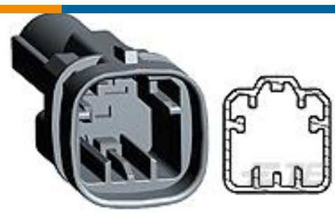
TE 系列/零件编号1544606-3 TAB HOUSING, 8MM NG1, 1 WAY
