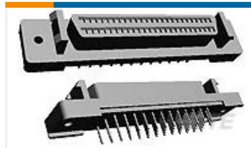
TE 系列/零件编号5786136-5 50 50SR VERT RCPT ASSY
