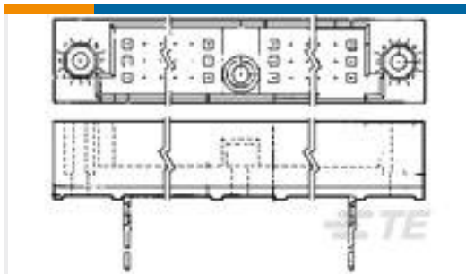
TE 系列/零件编号533294-1 HDI PIN ASSY 3 ROW 240 POS
