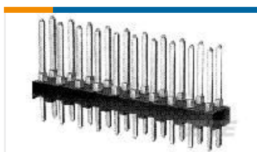
TE 系列/零件编号1-87215-2 06 MODII HDR DRST UNSHRD .100
