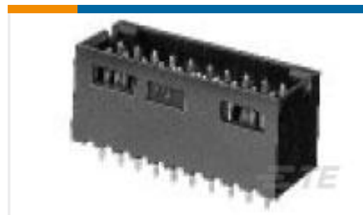
TE 系列/零件编号102618-8 20 MODII HDR DRST SHRD .100CL
