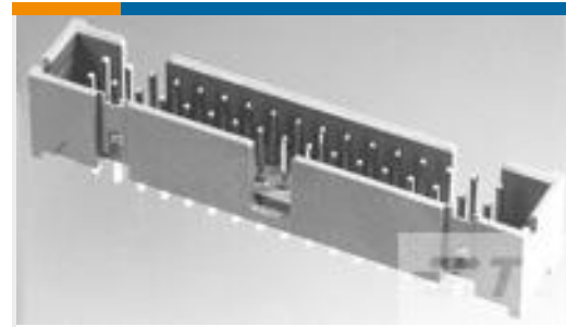
TE 系列/零件编号5104338-6 A/L LOW PRO HDR 26P VERT HT
