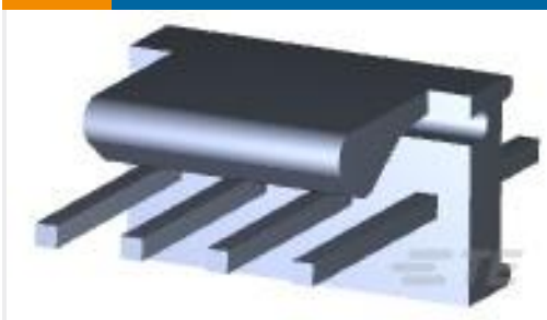
TE 系列/零件编号3-641126-4 04P MTA100 HDR ASY FL /STR LF
