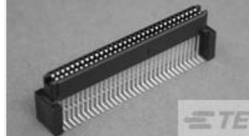
TE 系列/零件编号1-5146896-1 1FHR,64,50A/S,S,C,S14,15
