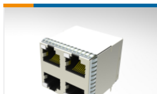
TE 系列/零件编号2303402-1 STK MJ ASSY,8POS,2X2, CAT5E
