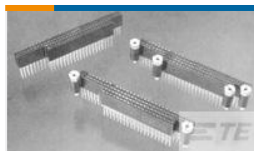
TE 系列/零件编号1375794-1 ASSY, 64/40 POS PC104
