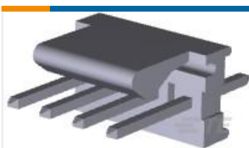
TE 系列/零件编号644518-4 04P MTA100 HDR ASSY FL STR SN
