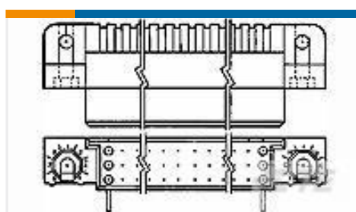
TE 系列/零件编号104361-2 03 MTE HDR SRRA LATCH W/HLDWN
