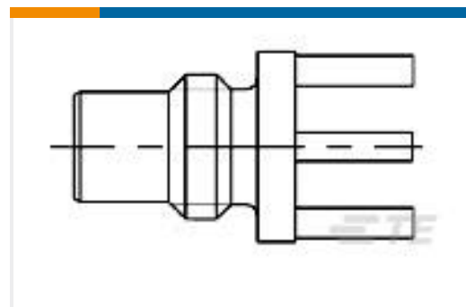
TE 系列/零件编号1060256-1 5062 5003 09,SMC PCB JACK RECP
