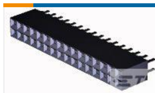
TE 系列/零件编号1-146762-8 32 MODII RCPT VERT DR
