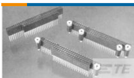
TE 系列/零件编号1375963-2 PC104 CONN NONSTKTHRU NO STNDO
