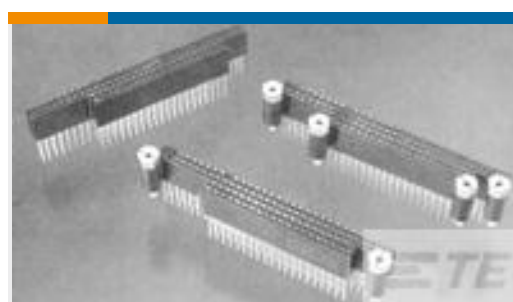
TE 系列/零件编号1375963-2 PC104 CONN NONSTKTHRU NO STNDOL
