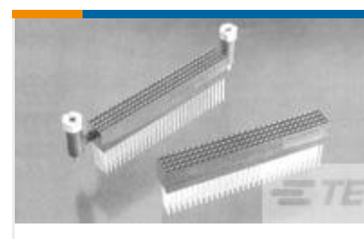
TE 系列/零件编号1375800-1 ASSY, 120 POS PC104 PLUS
