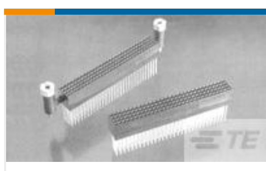
TE 系列/零件编号1375800-4 ASSY, 120 POS PC104 PLUS LF
