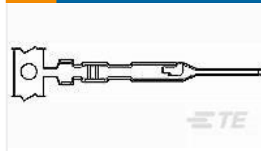
TE 系列/零件编号1-104506-0 MTE PIN 28-32 AWG PLTD
