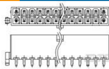
TE 系列/零件编号1- 1775099-3 ATX PWR CONN 1 BDLK 24 POS
