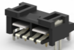
TE 系列/零件编号1982295-1 ELCON MINI 2P RA HEADER, W/CODING
