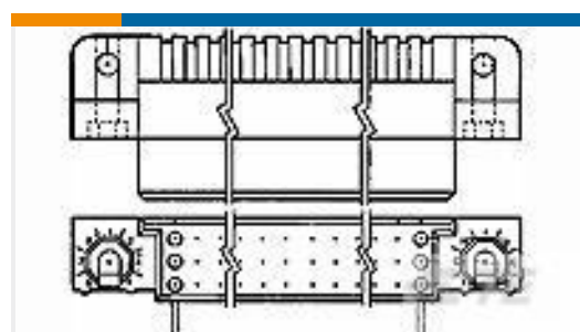
TE 系列/零件编号533268-6 HDI RECP ASSY 3 ROW 135 POS
