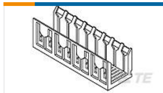
TE 系列/零件编号536565-3 2MMFB,SHRD,096,SIG, HDR
