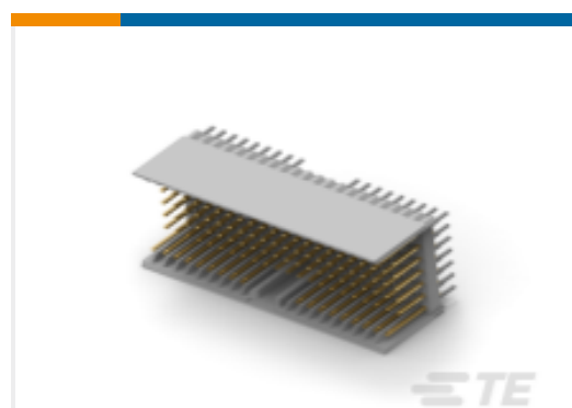
TE 系列/零件编号 5646533-1 2MM HM,TYPE A/B,HDR, ASY,146POS
