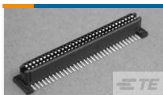
TE 系列/零件编号120521-1 1FHR,64,30A/P,S,N,S08, 09,10
