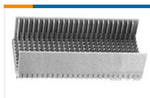
TE 系列/零件编号5646357-1 2MM HM ASY,T-B,HDR, 10R,250,AP
