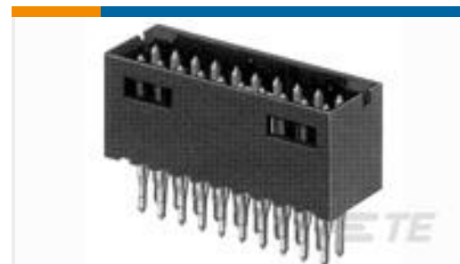
TE 系列/零件编号1-102557-1 08 MODII HDR DRST SHRD A/PIN
