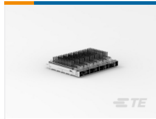
TE 系列/零件编号 2170747-6 CAGE ASSY, 1X4, QSFP28, SPRING, HS, LP
