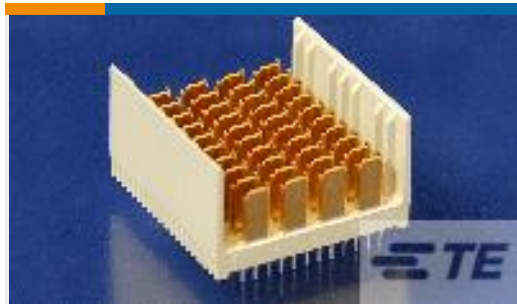
TE 系列/零件编号1469002-1 HM-ZD 4PR HDR 80P 5.2 MM
