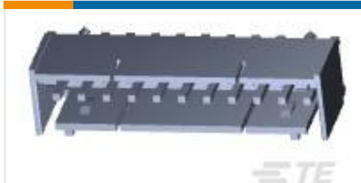
TE 系列/零件编号1-5646513-9 2MM H.M. 8 + 2 ROW TYPE "F" PI
