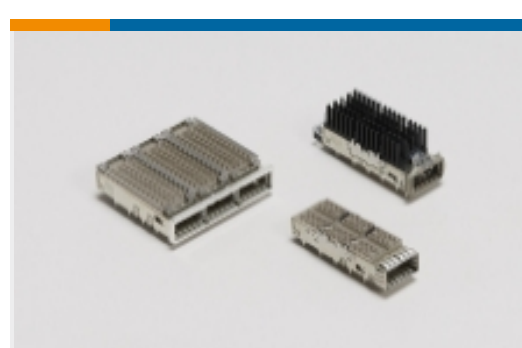
QSFP/QSFP+/zQSFP+(411)
