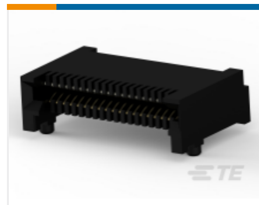
TE 系列/零件编号 2110819-1 QSFP+ Enh EVERCLEAR PT Conn
